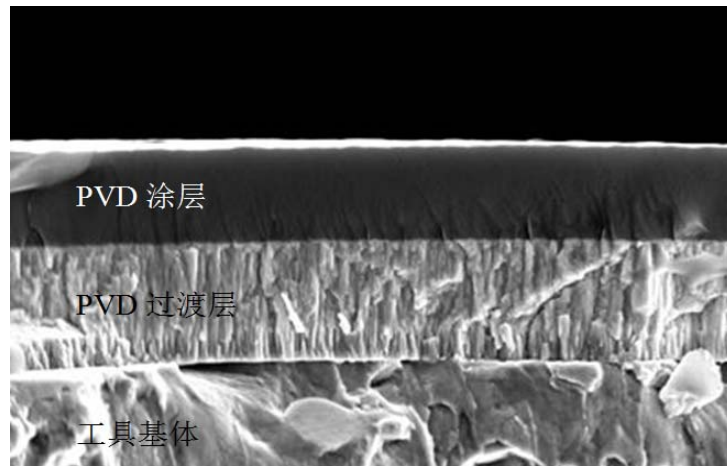
(图 2 PVD 涂层截面图)
